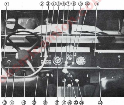
Fig. 4. Mandos, instrumentos e indicadores (Mod. L.)
