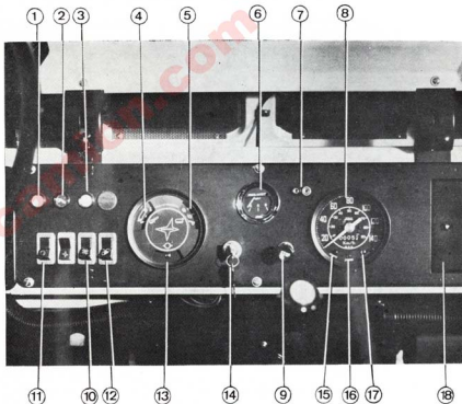
Fig. 6. Mandos, instrumentos e indicadores (Mod. L.)
