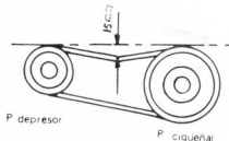
Fig. 75. Flexión máxima de la correa del depresor.
